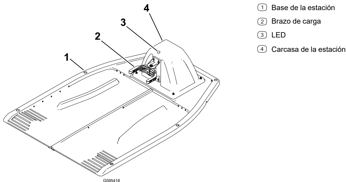
Figura 4 Componentes de la estación de carga
