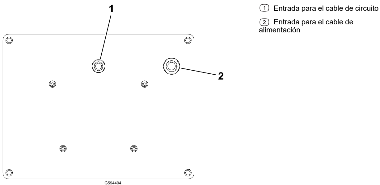
Figura 5 Vista inferior de la base de la estación
