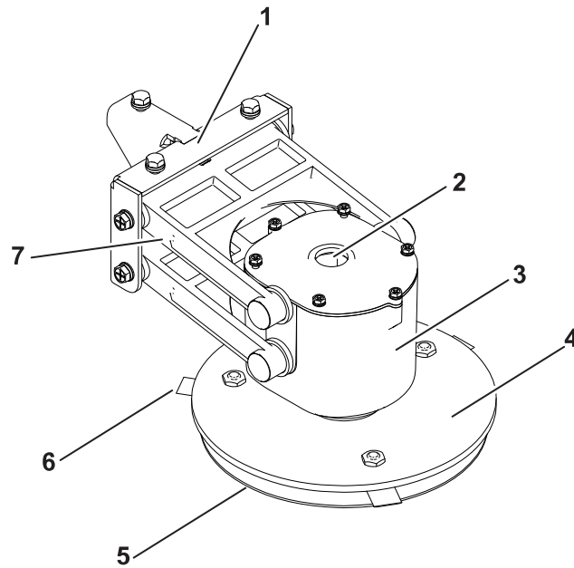
Figura 3 Cabezal de corte
