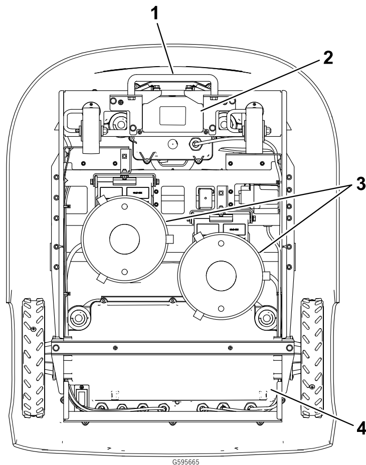
図 1 底面図
