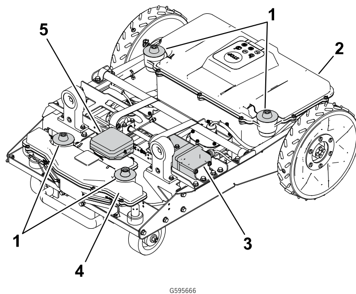
図 2 上面図（シェルを取り外した状態）
