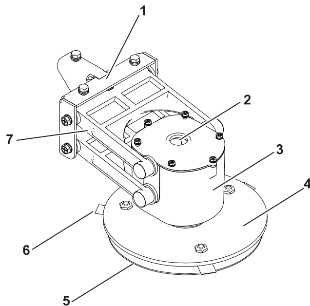
図 3 カuttingヘッド
