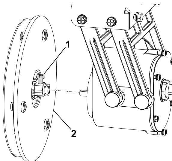
① 固定ねじ
