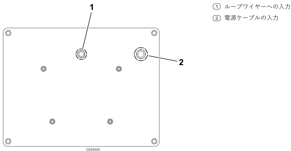
図 5 ステーションベースの底面図
