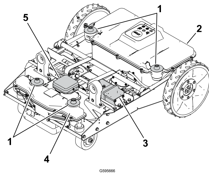
Figur 2 Sett ovenfra (skallet fjernet)
