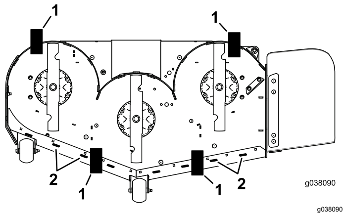
Figur 84 Sett nedenfra
