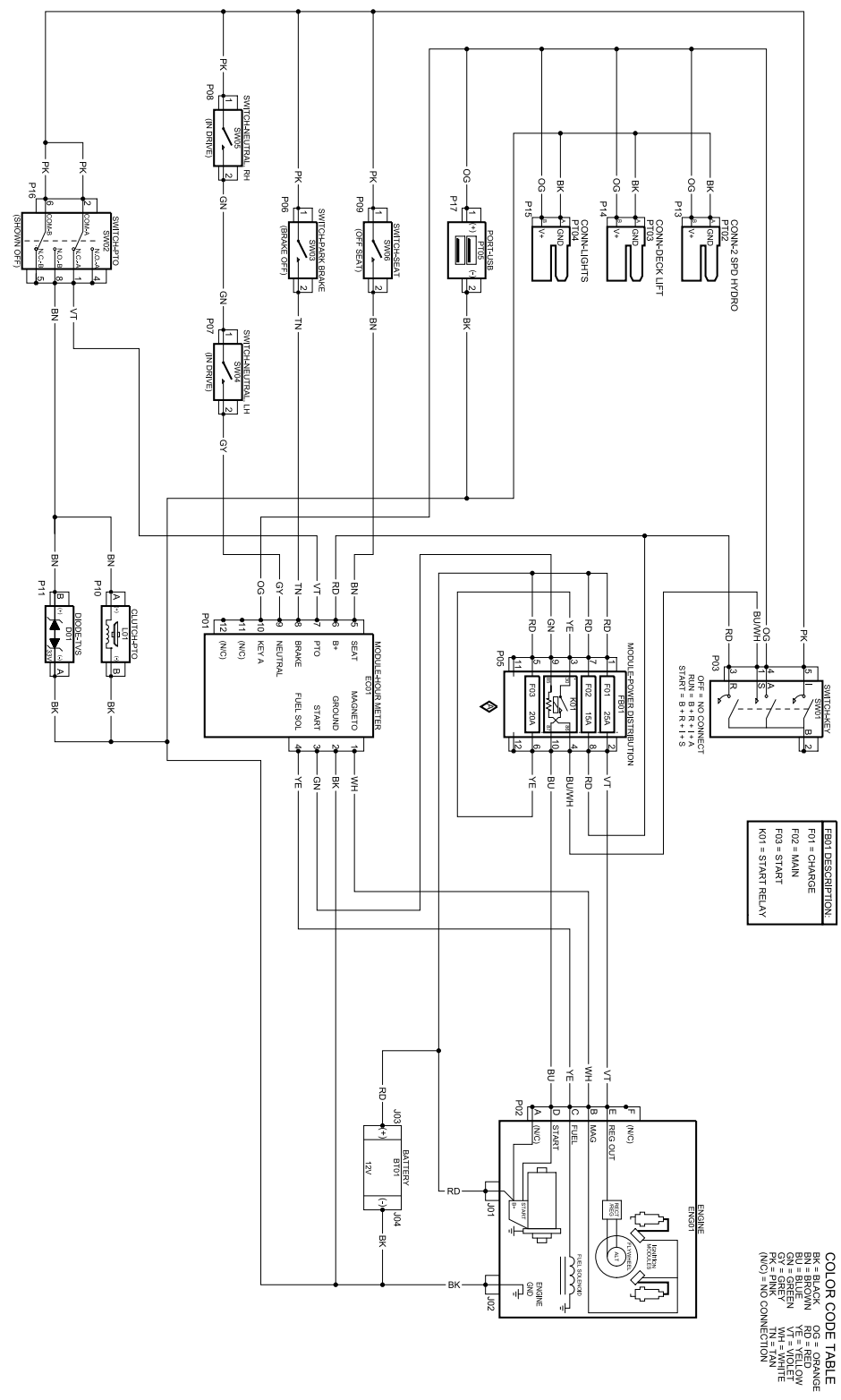
Schema elettrico – pagina 1 (Rev. A)
