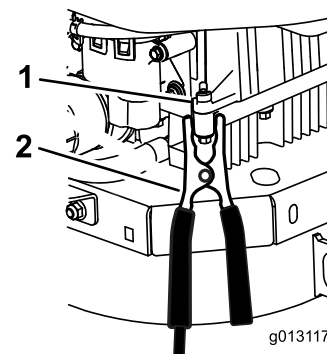
1. Bloque motor 2. Cable negativo (-)
