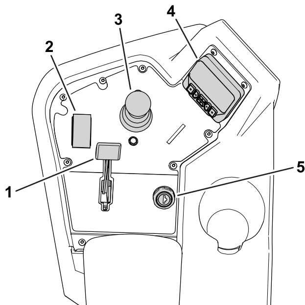
Kuva 18 Kojetaulu
