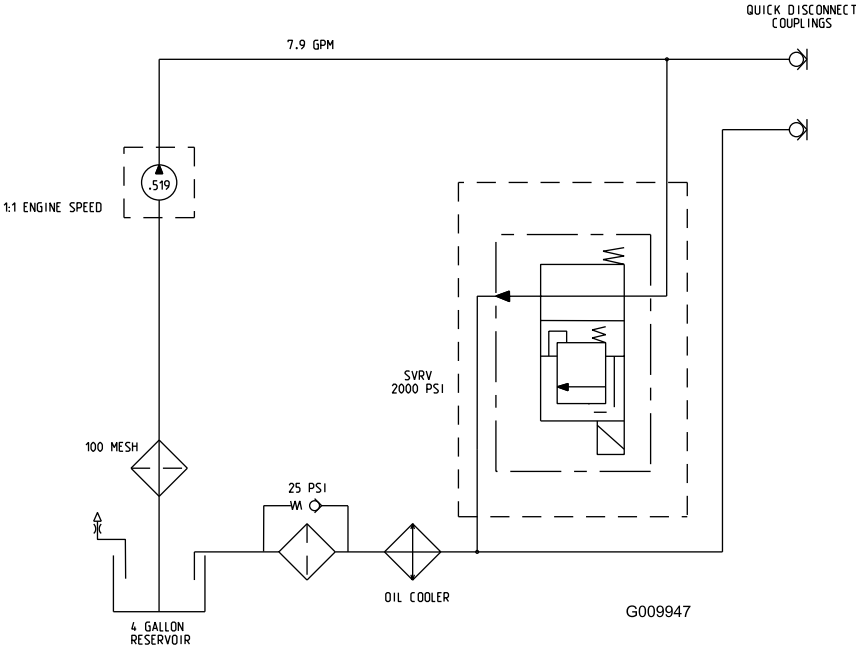
Hydraulikaavio (Rev. A)
