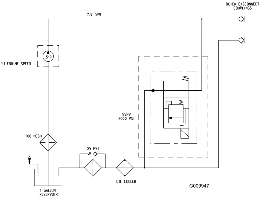
Hydraulikkskjema (Rev. A)
