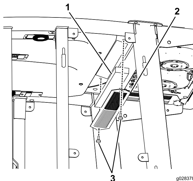
Figuur 148 Luchtfiler in de cabine
