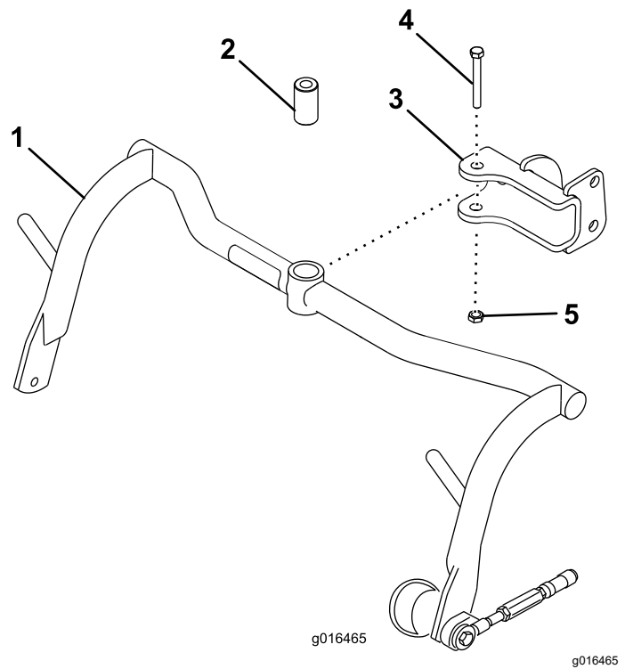
Figur 6
