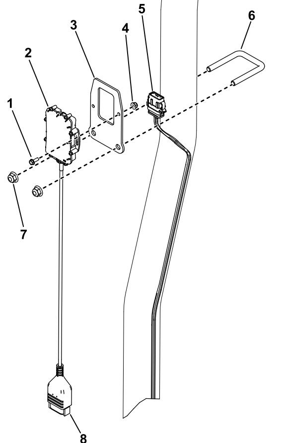
Figur 5
