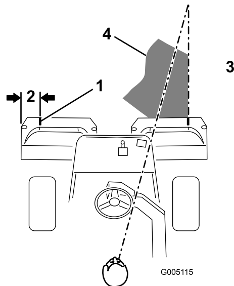
Figur 10
