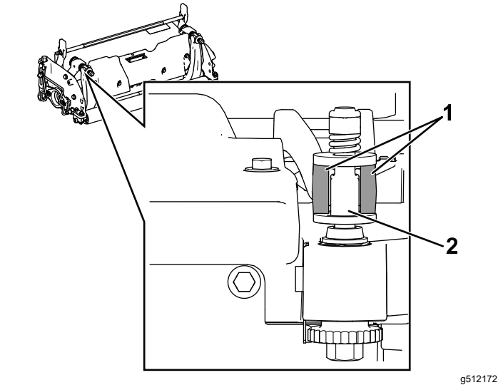
图 21
