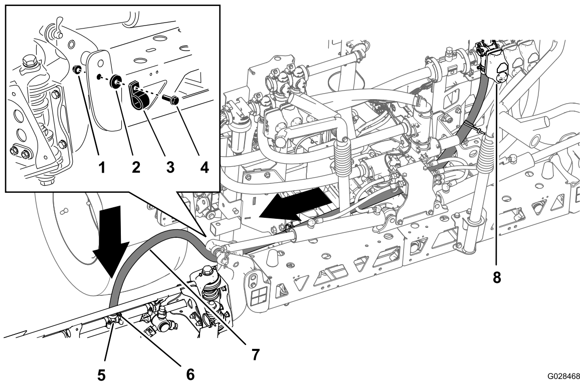
Figura 40 Manguera – Sección de brazo izquierda
