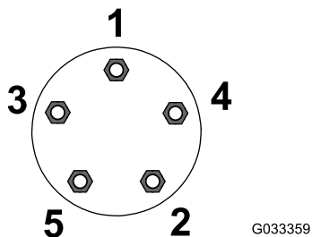
Figura 17 Ruedas traseras
