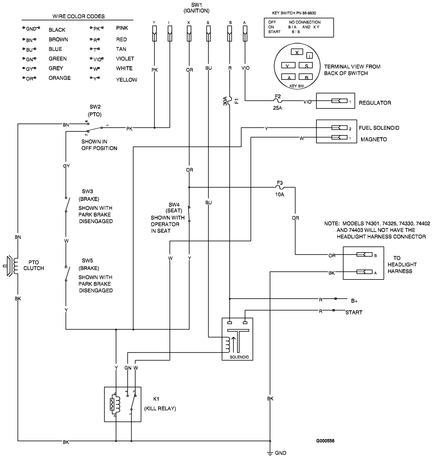
Schéma électrique (Rev. A)
