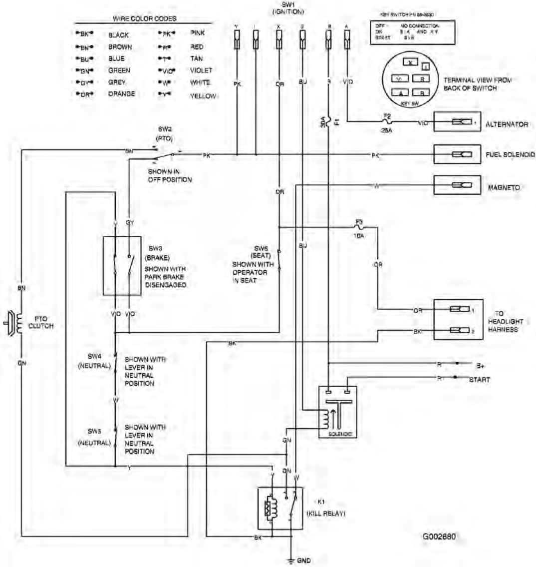
Ledningsdiagram (Rev. B)
