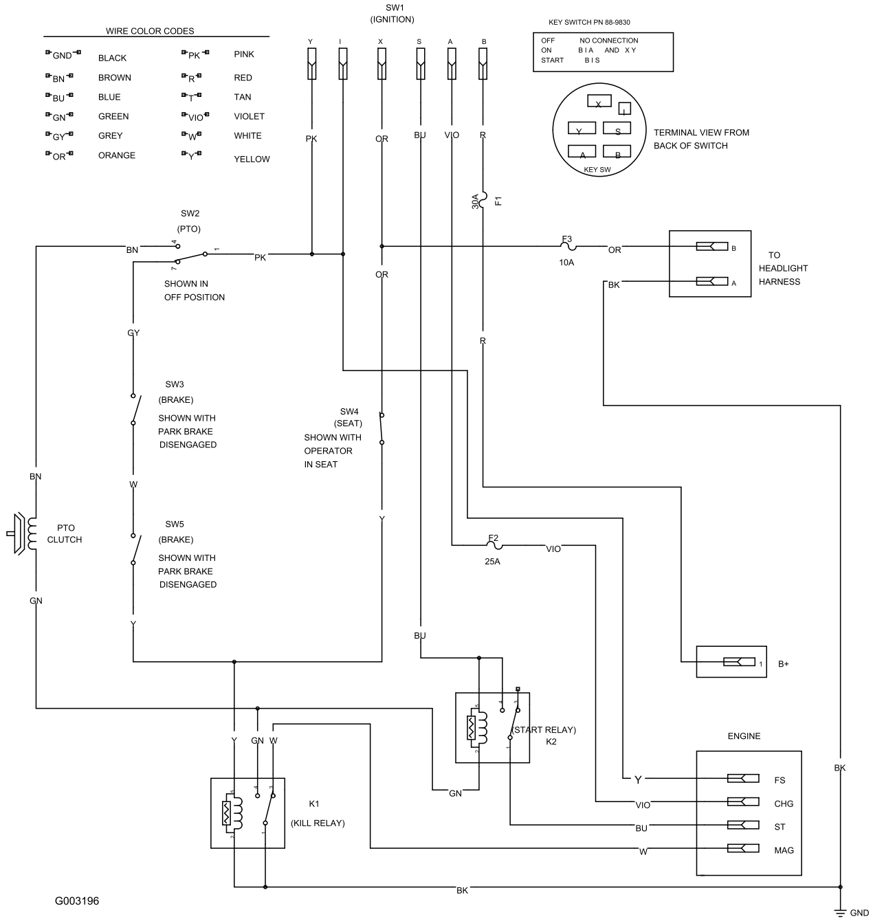
Installatieschema (Rev. B)
