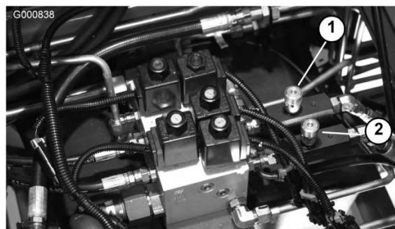
Figura 75 Modelli 03806 e 03807
