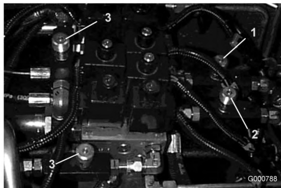
Figura 74 Modello 03808
