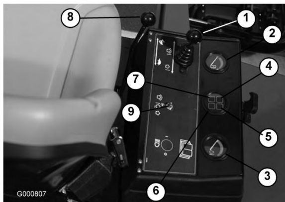
Figura 11 Modelos 03806 e 03807
