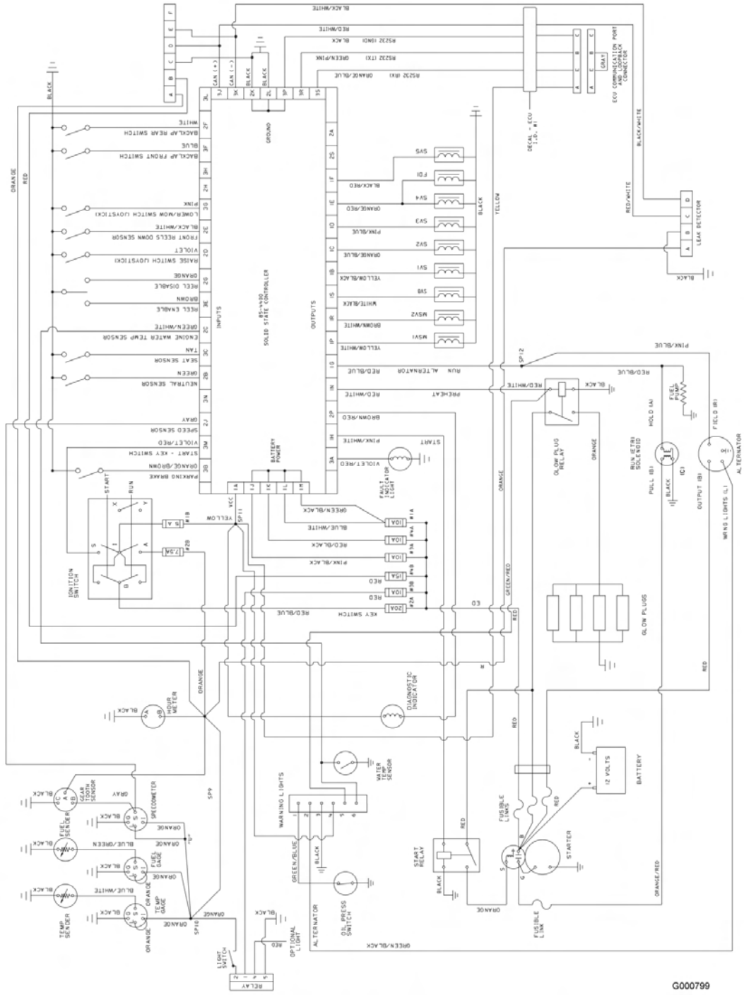
Elschema (Rev. -)
