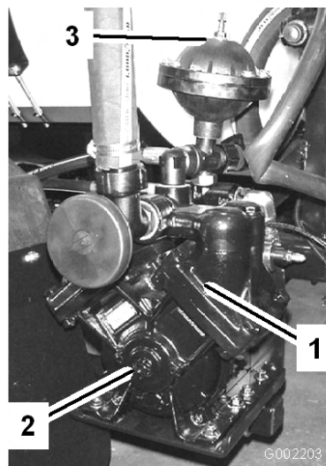
1. Bomba 2. Punto de engrase 3. Amortiguador de presión
