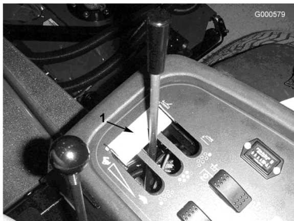
Figure 11 Modèle 4500-D
