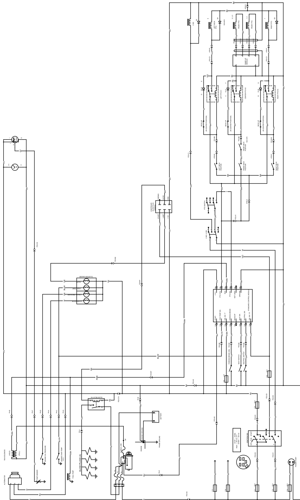
Schéma électrique (Rev. C)
