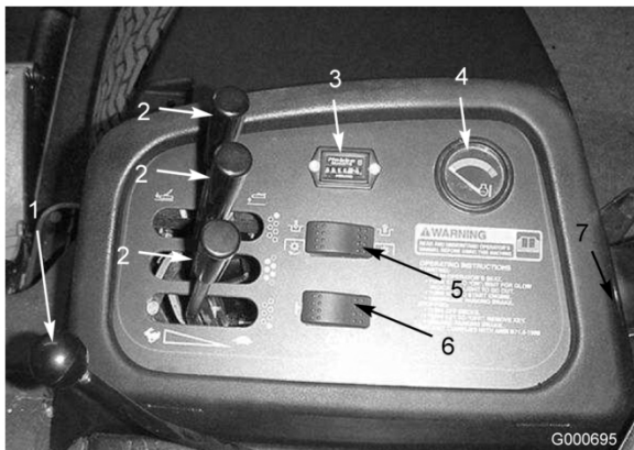
Figure 9 Modèle 4700-D
