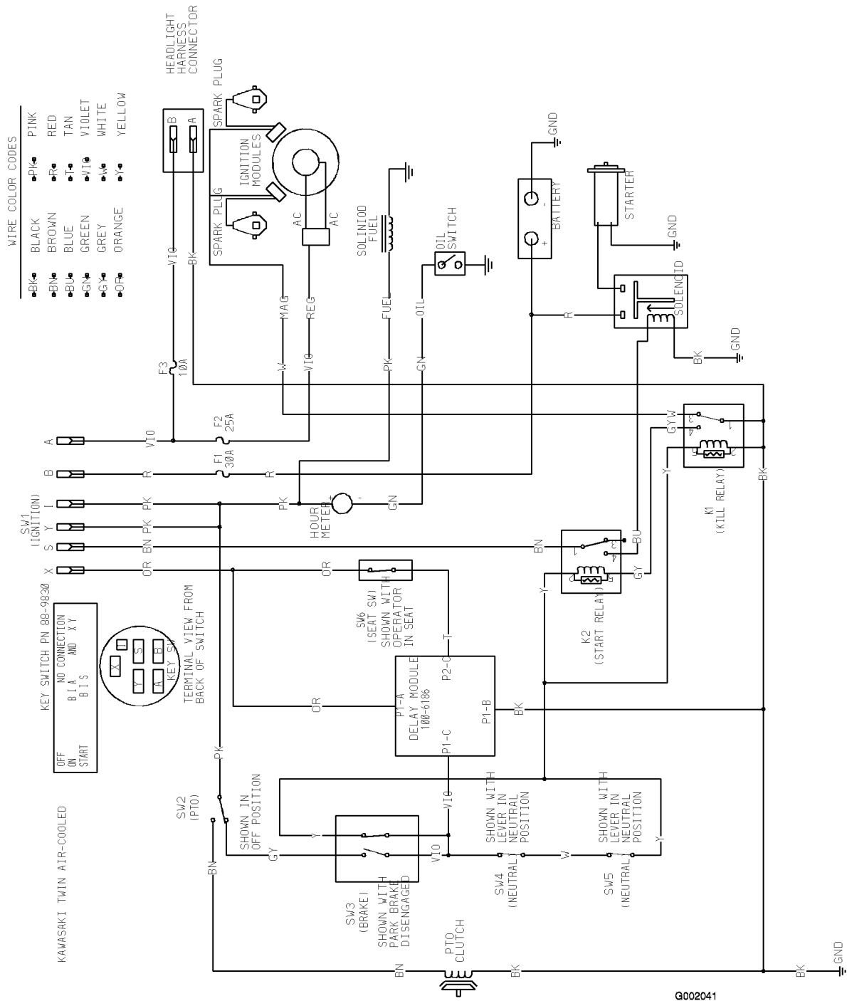
Schéma de câblage (Rev. A)
