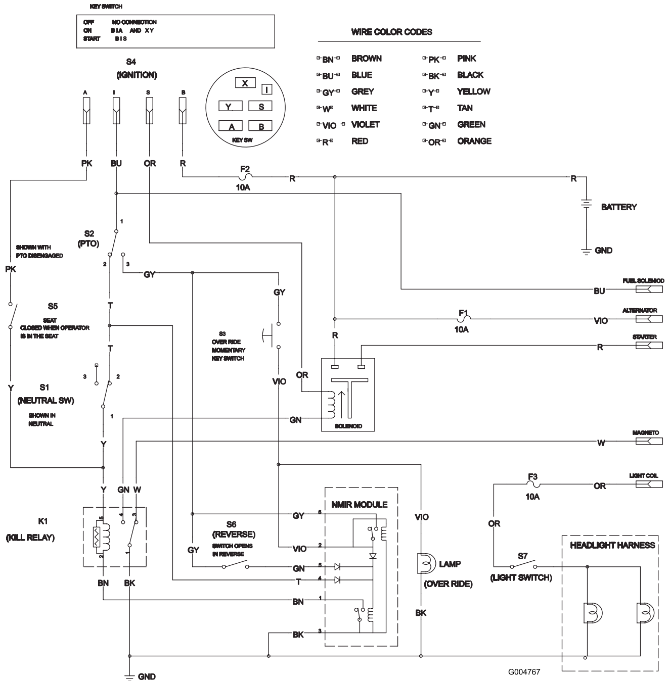
Schaltbild (Rev. A)
