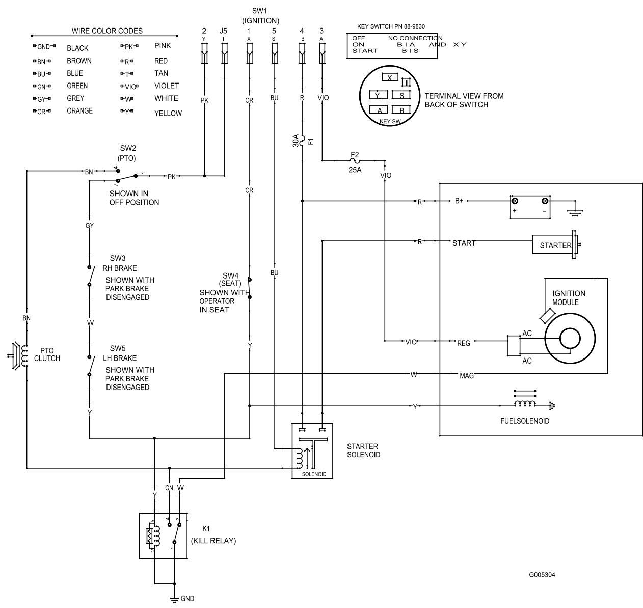
Installatieschema (Rev. A)
