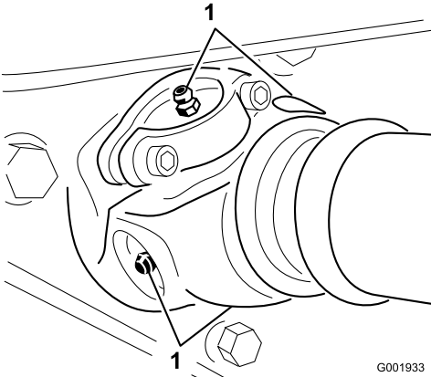
Figure 38 Entraînement de pompe, quatre de chaque côté
