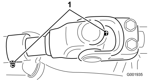
Figure 40 Essieu moteur à transmission, cinq de chaque côté
