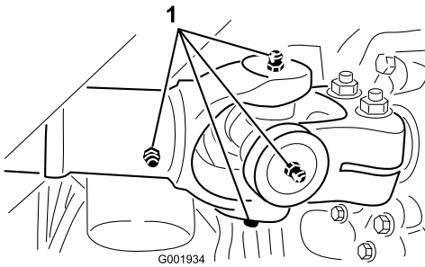
Figure 39 Essieu moteur au moteur, cinq de chaque côté
