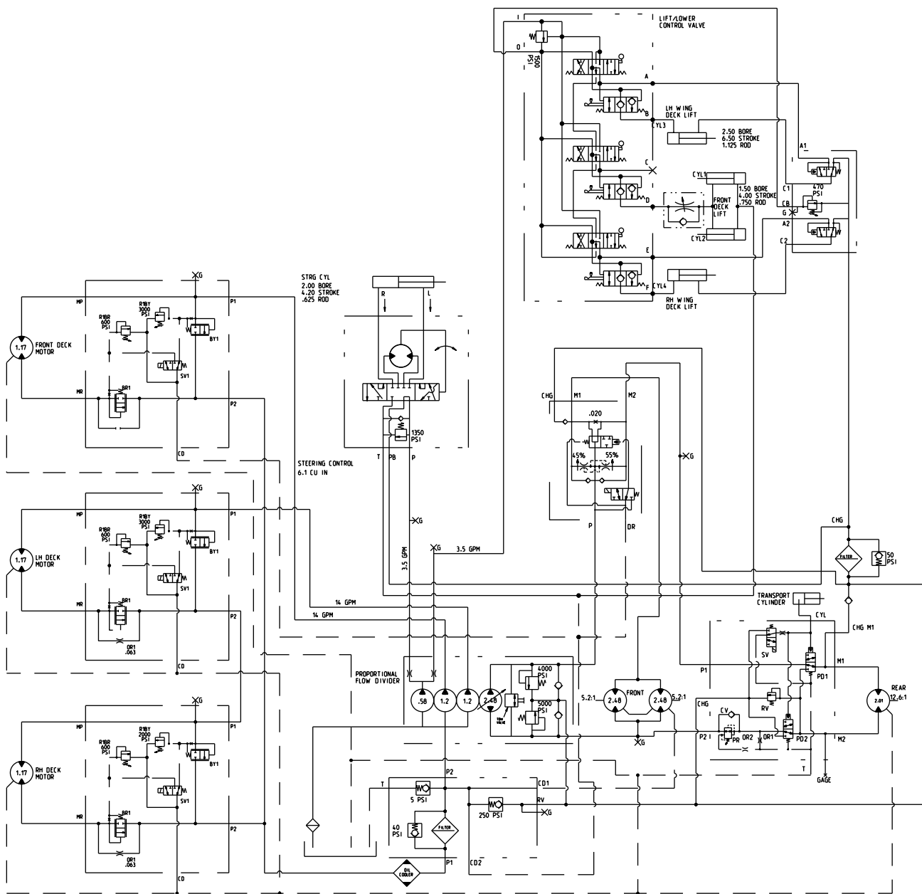
Schéma hydraulique (Rev. F)
