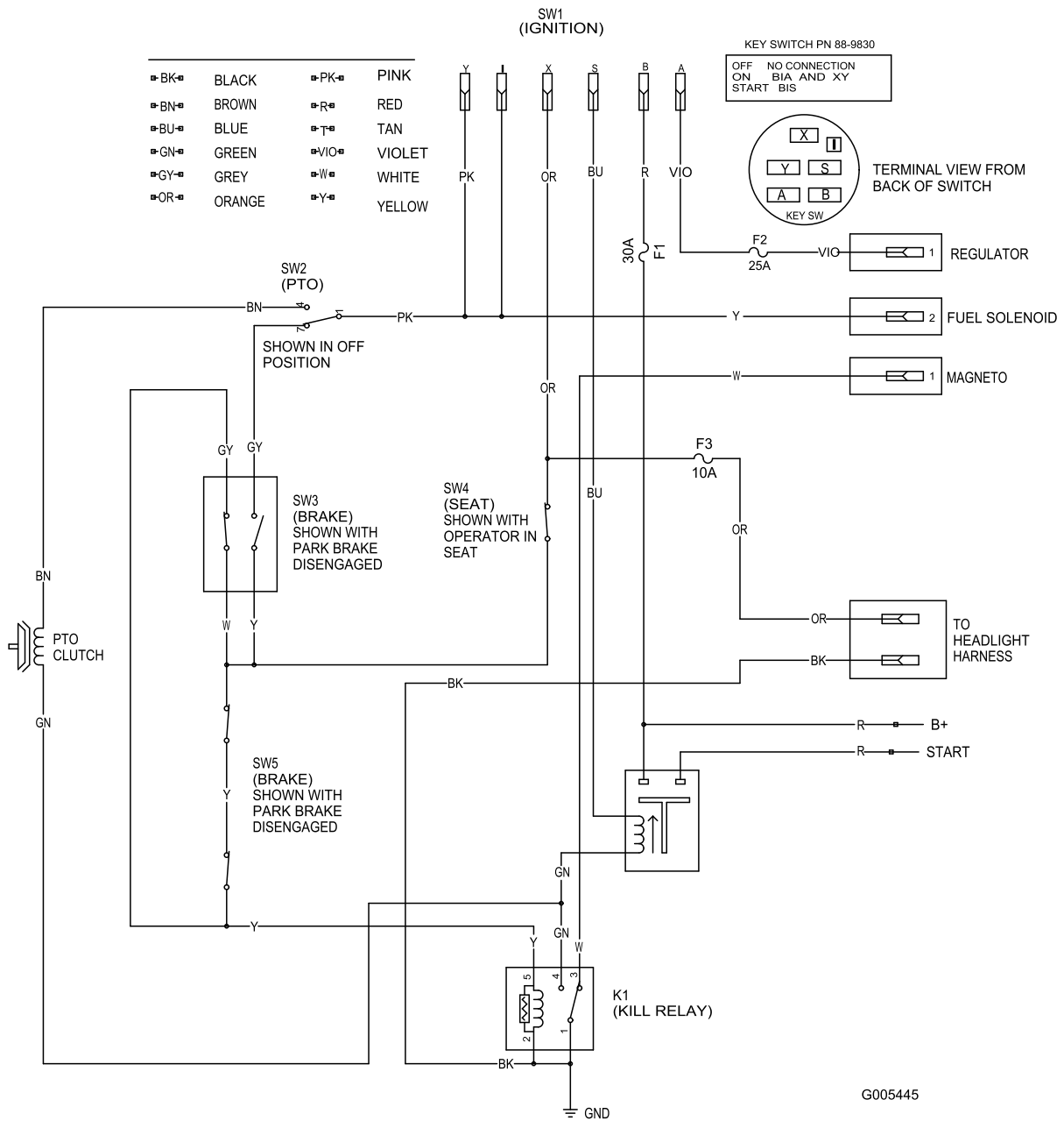
Schema elettrico (Rev. C)
