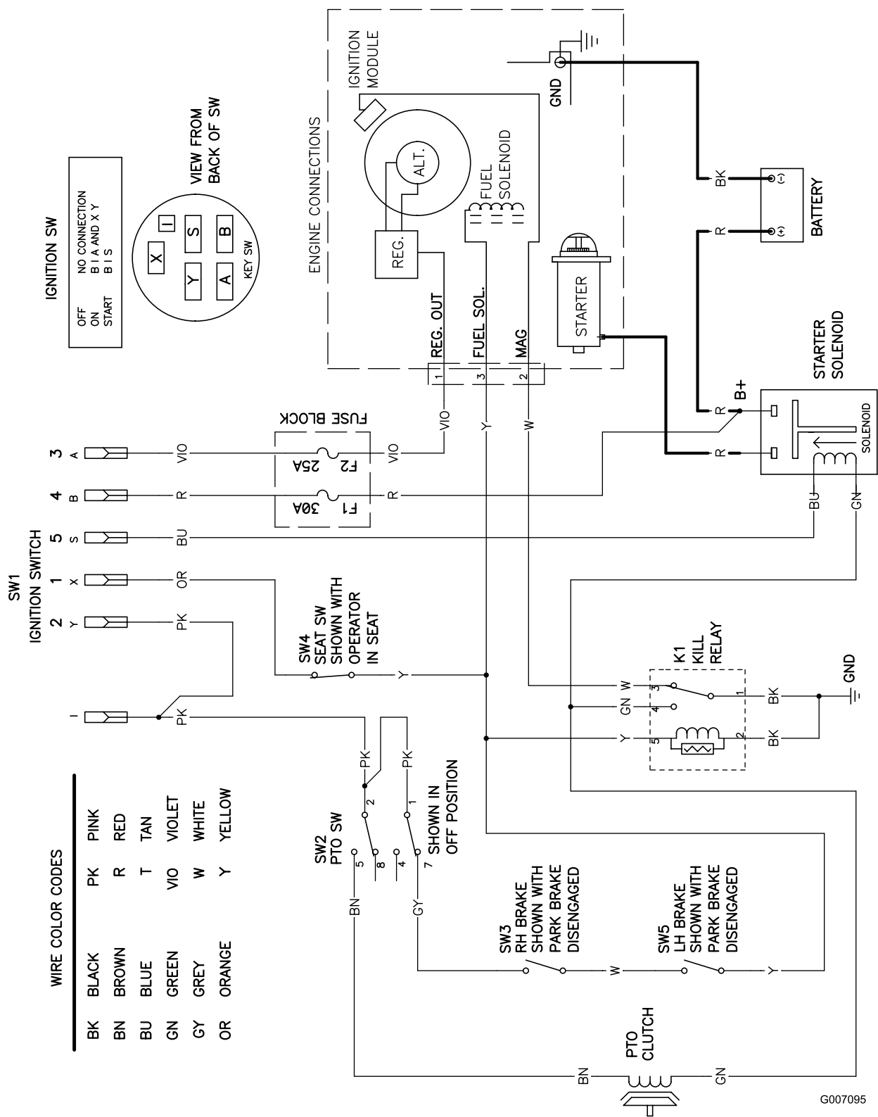
Koblingsskjema (Rev. A)
