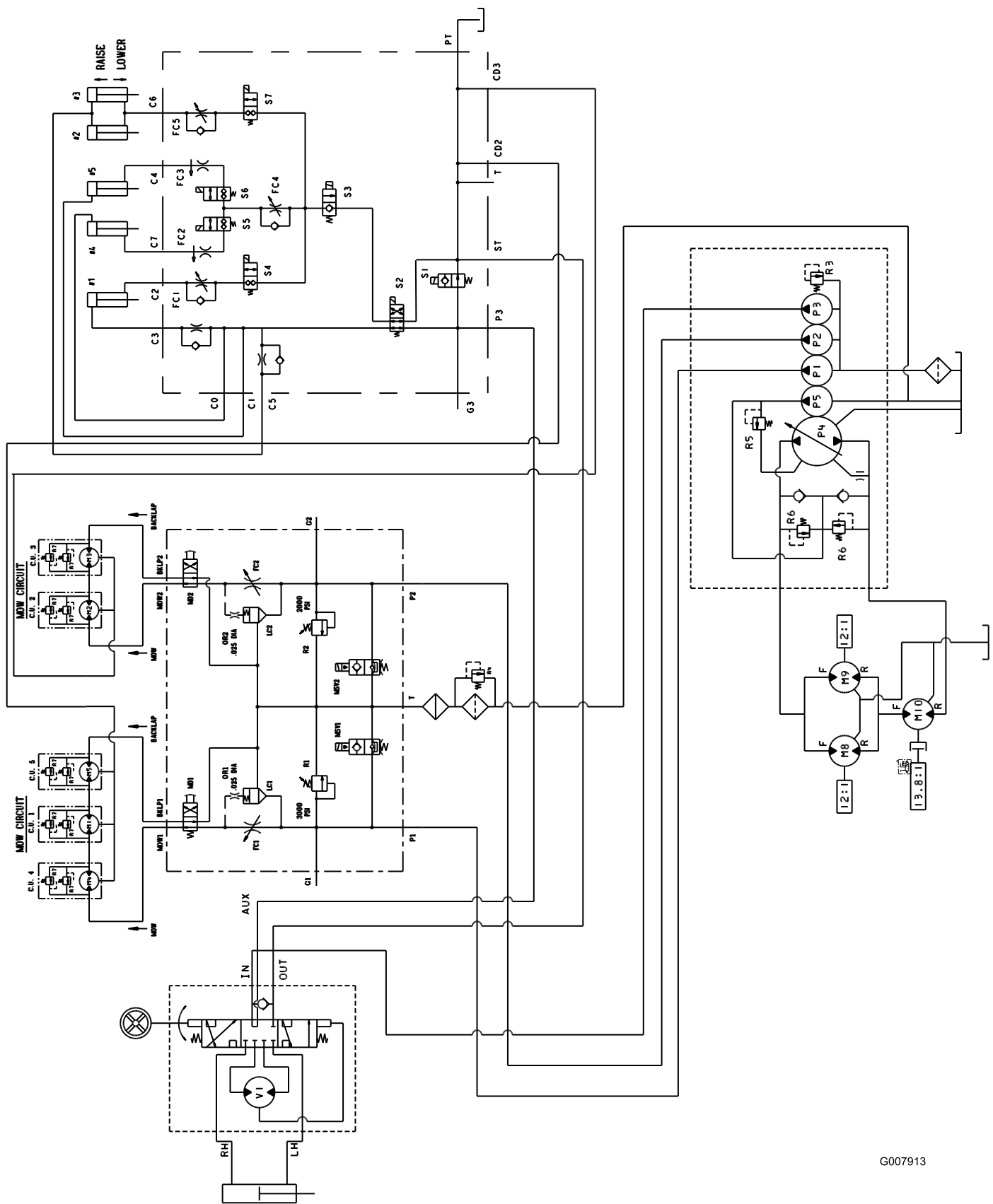
Schéma hydraulique, Modèle 03807 (Rev. -)
