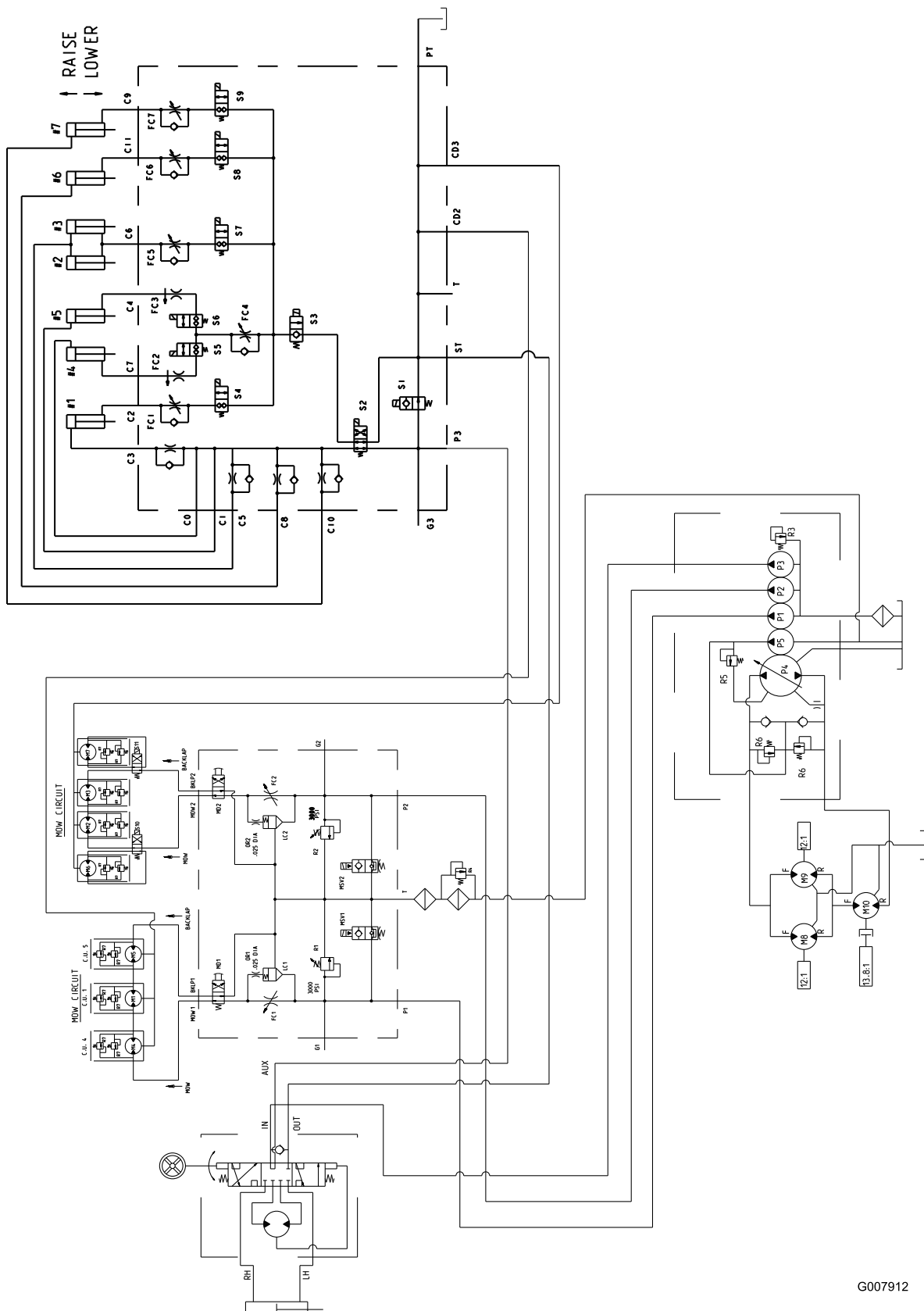
Schema idraulico del modello 03808 (Rev. A)
