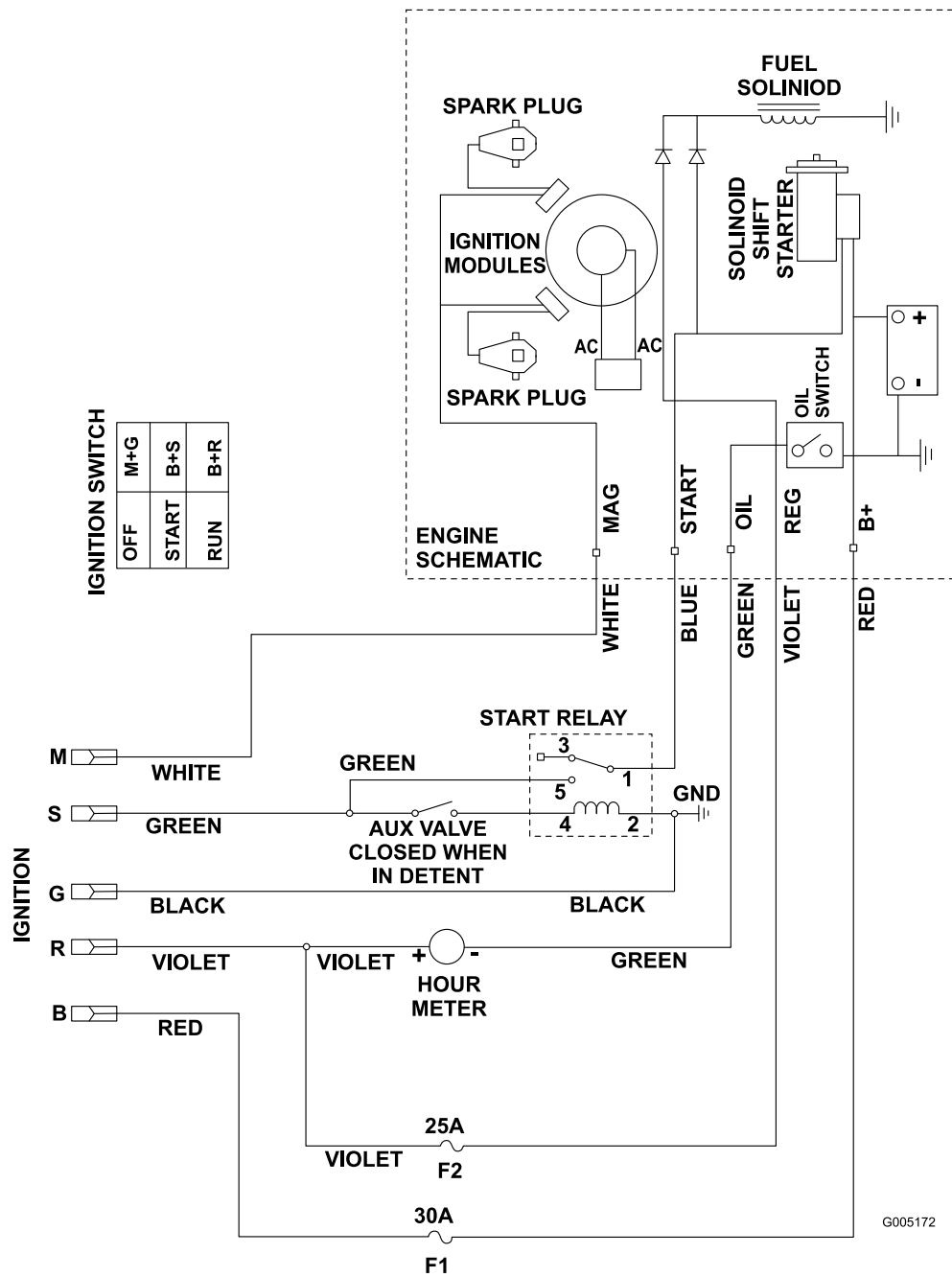
Schéma électrique (Rev. A)
