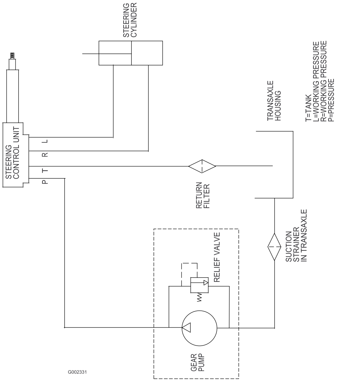
Hydraulikaavio (Rev. -)
