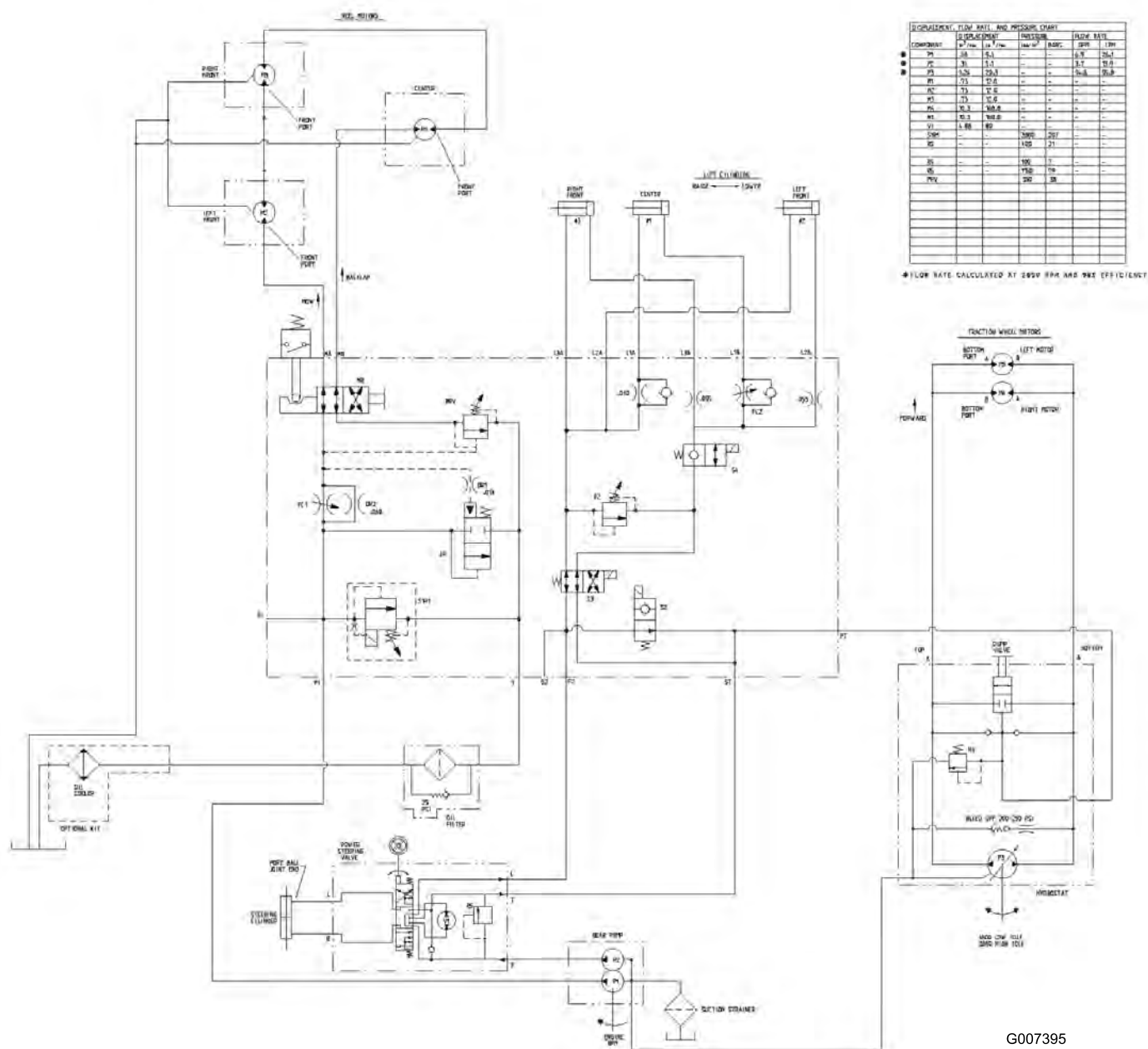
油压回路图 (Rev. A)
