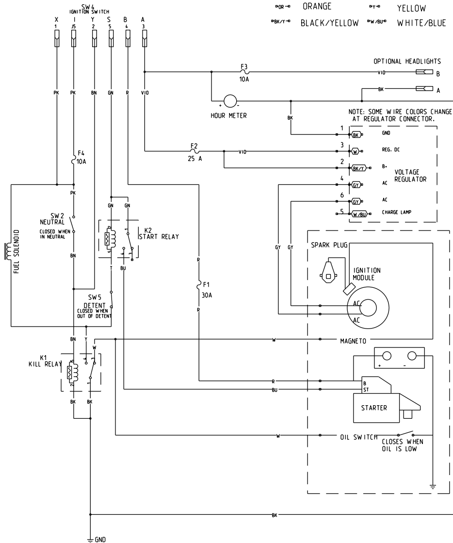
Esquema eléctrico (Rev. A)
