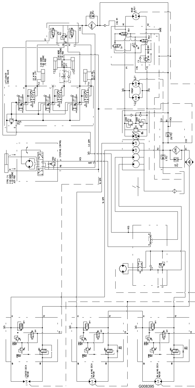
Esquema hidráulico (Rev. A)
