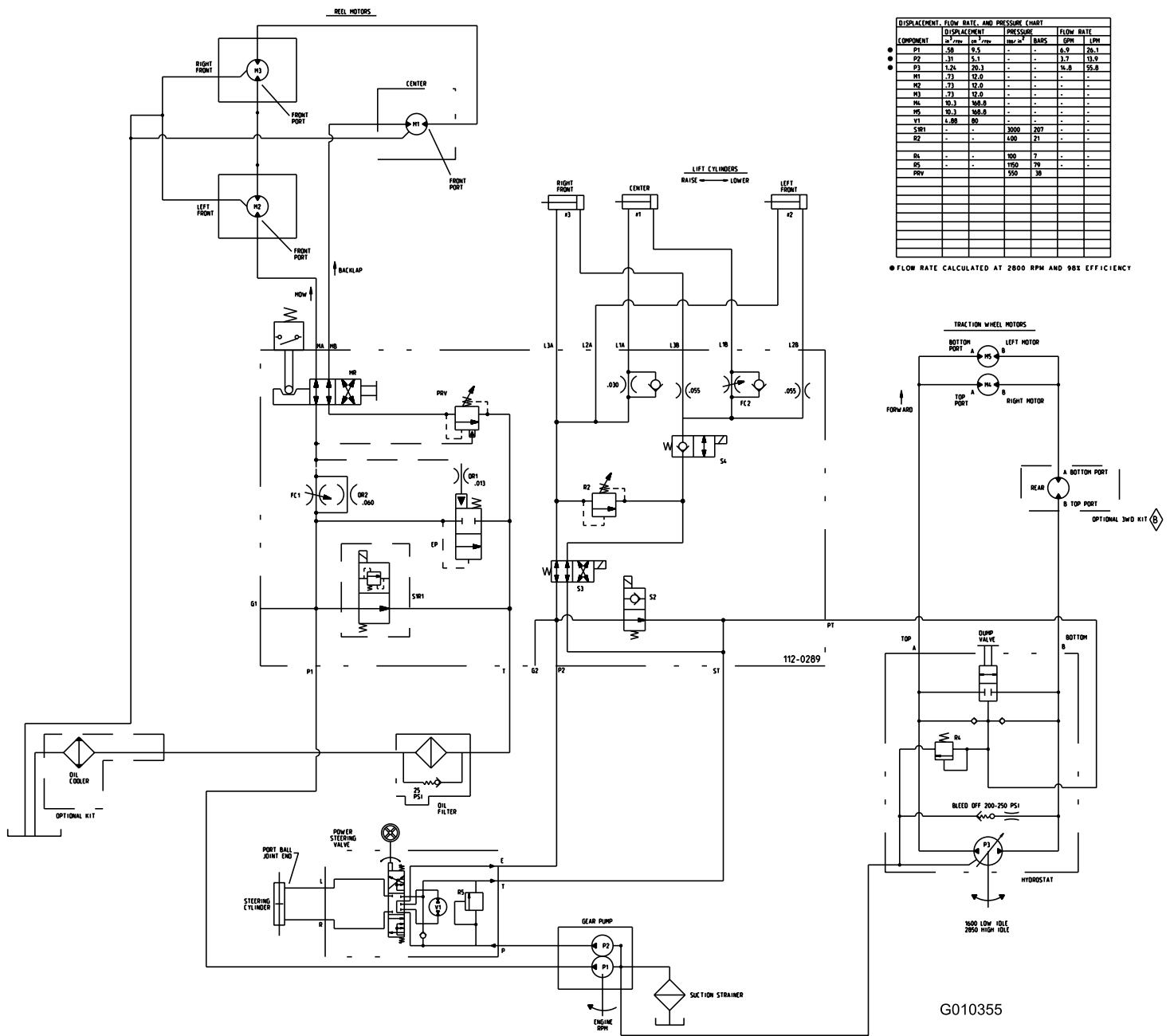
Hydraulisch schema (Rev. A)
