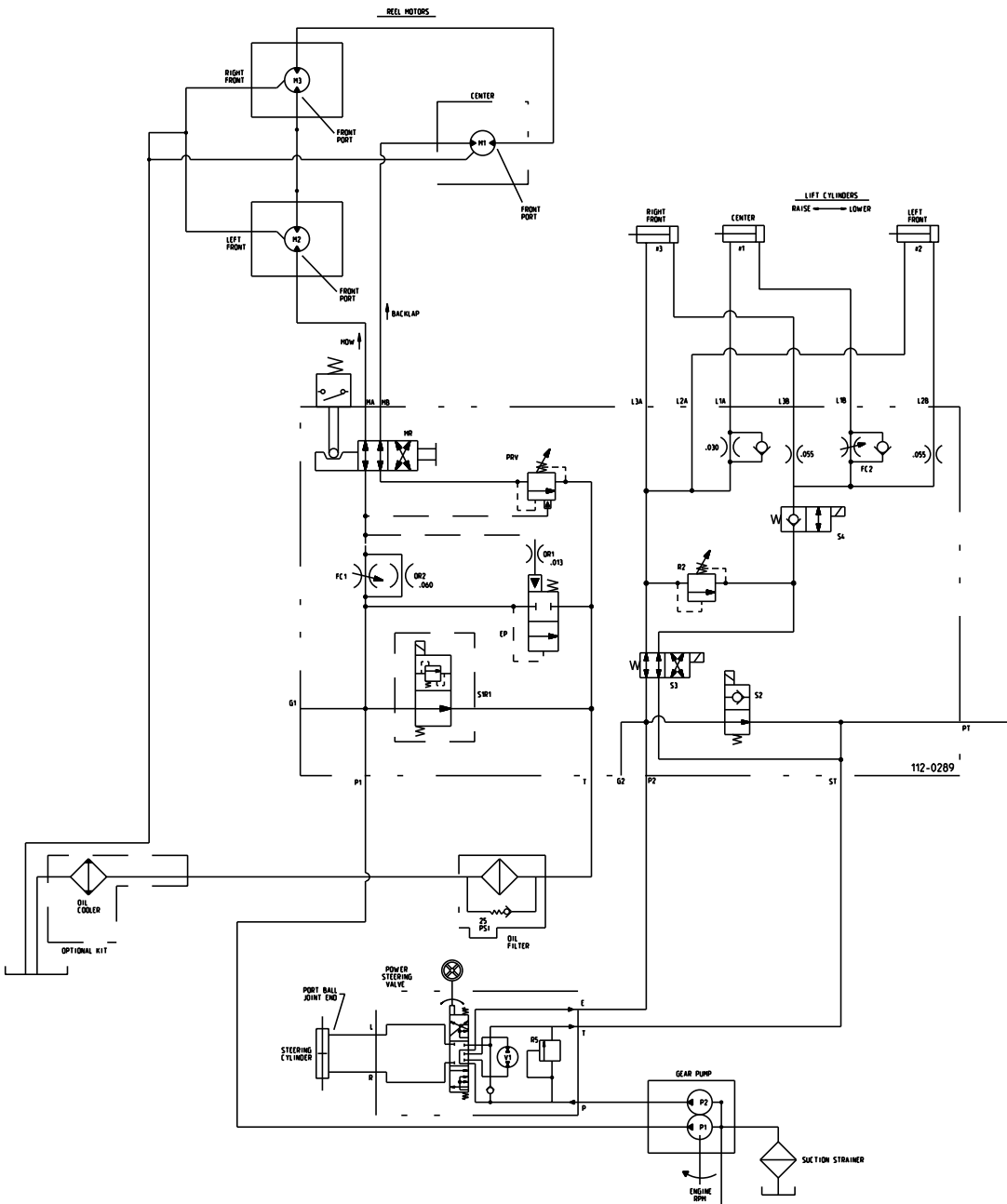
Hydraulikkskjema (Rev. A)
