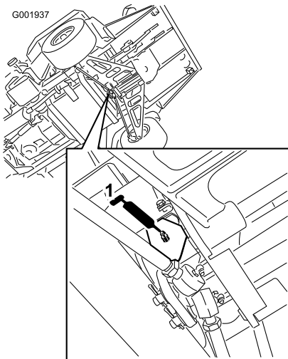
Figur 42 Styretap over styrestænger
