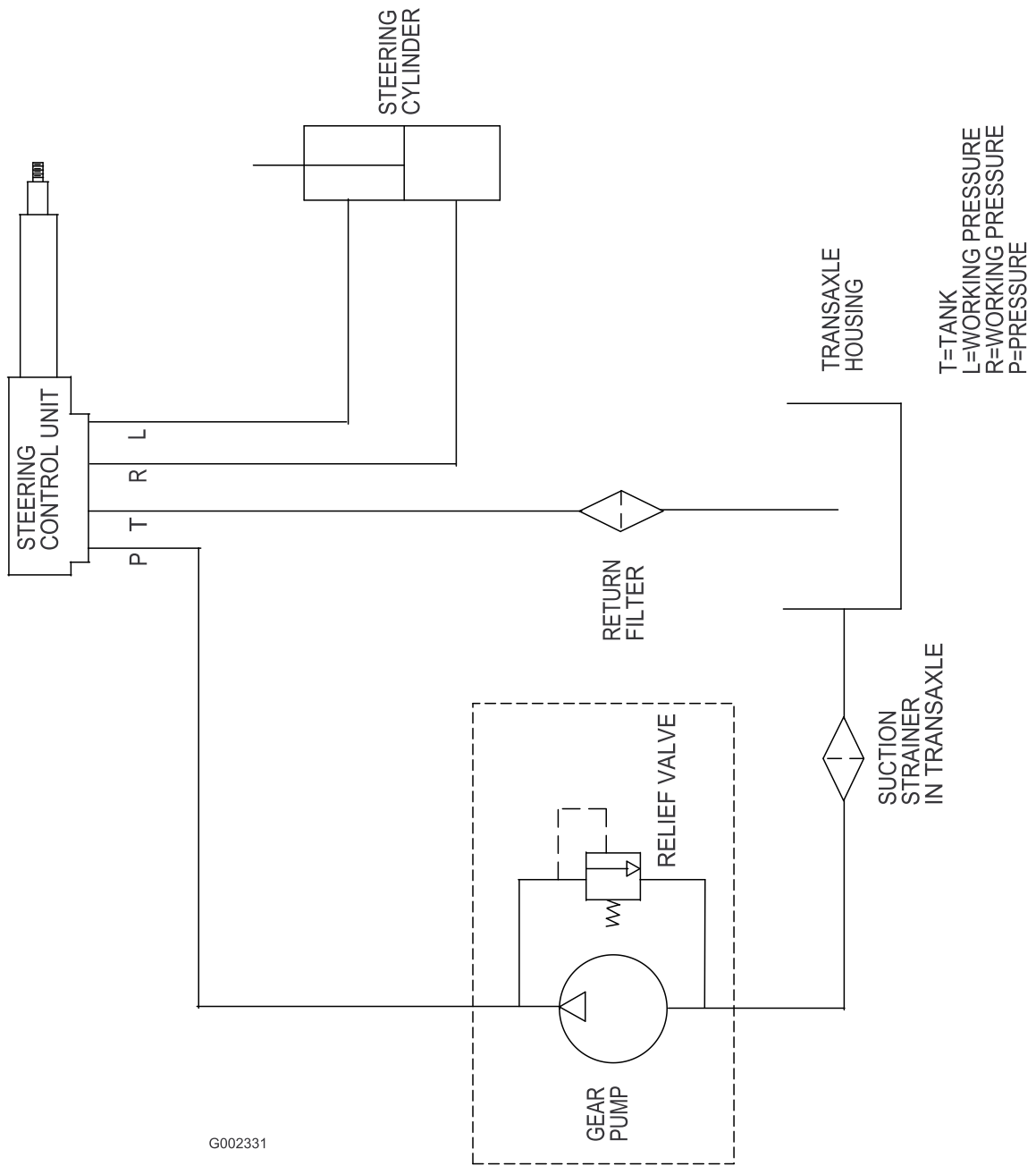
Hydrauliikk skjema (Rev. -)
