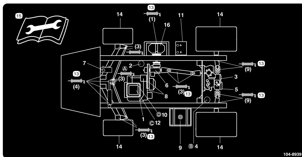
図 32 整備箇所
