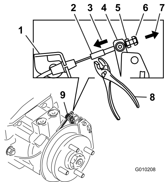
Figure 71 Frein gauche illustré
