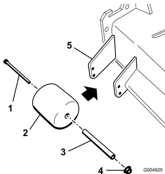
Bild 30 Nur Seitenauswurf-Mähwerke
