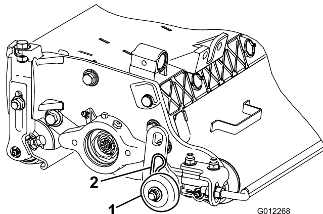
1. Transportrullenhet 2. Saxpinne
