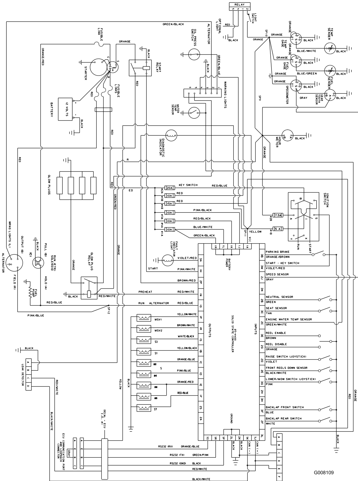
電気回路図, 全モデル (Rev. A)
