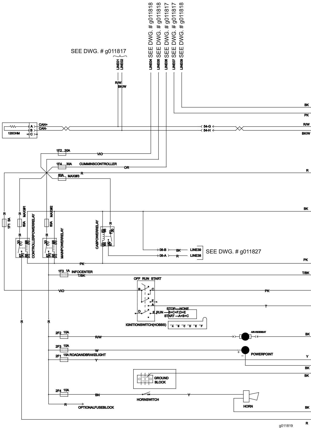
Schéma électrique (G011819) (Rev. A)
