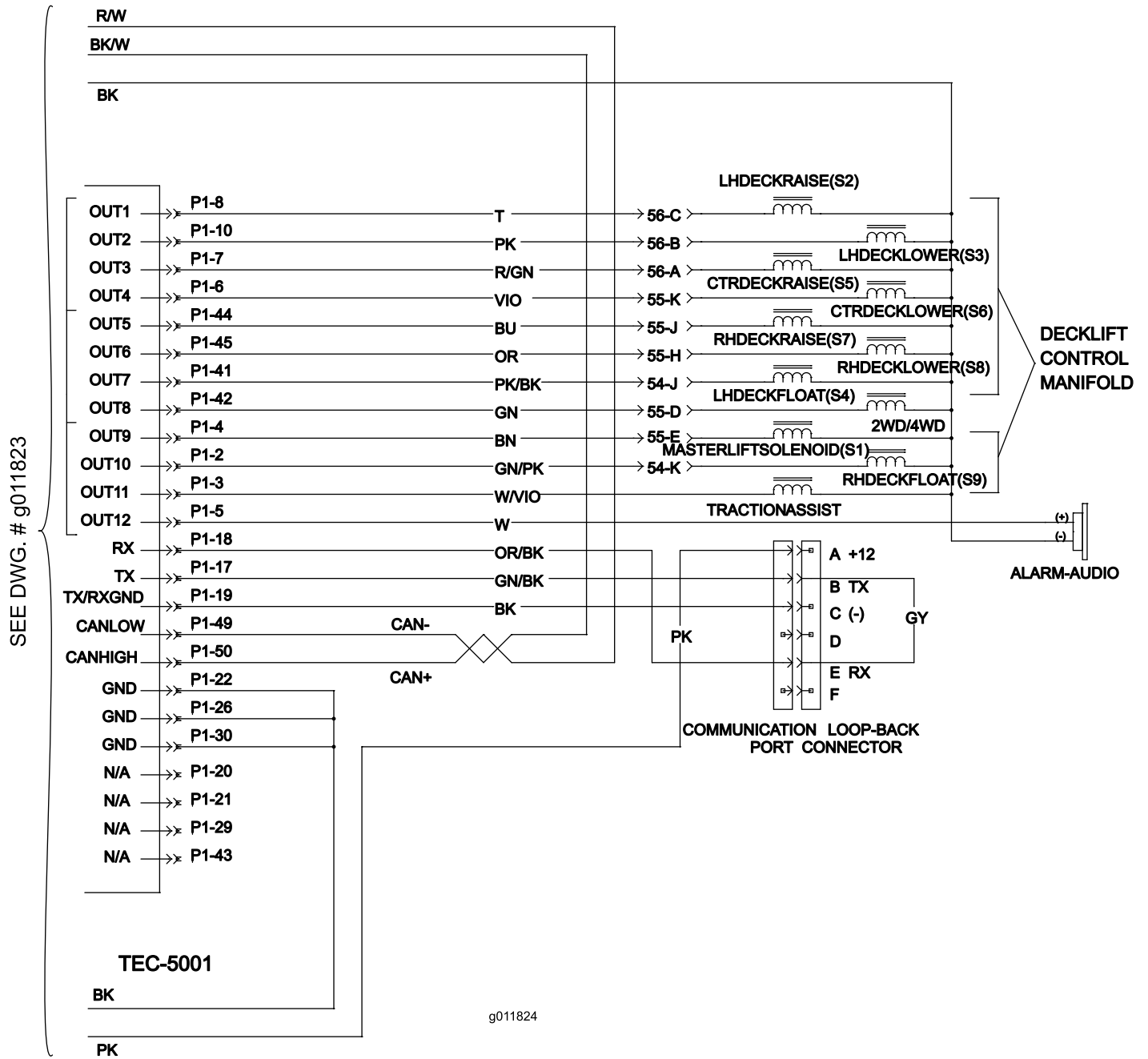
Elschema (G011824) (Rev. A)
