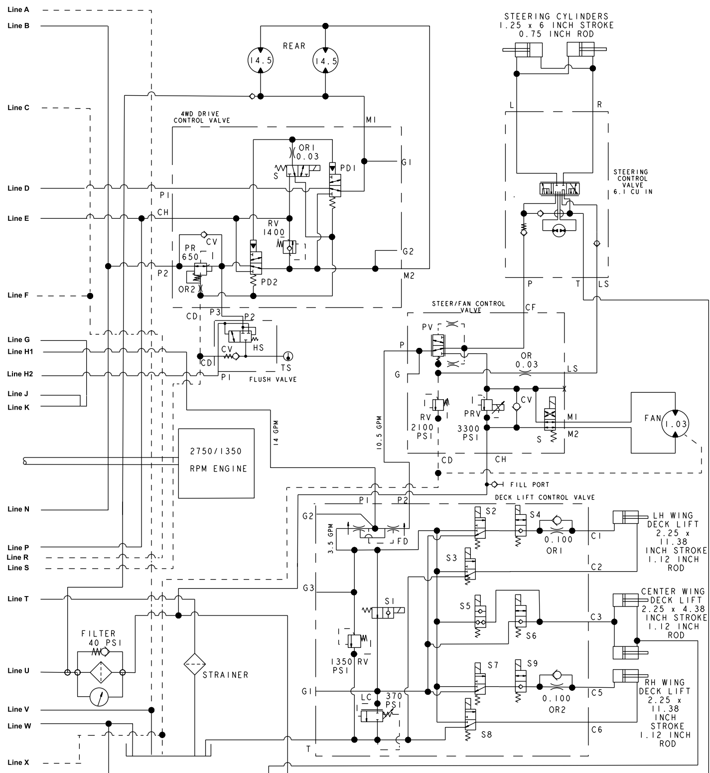
Hydraulschema (sidan 2 av 2) (Rev. A)
