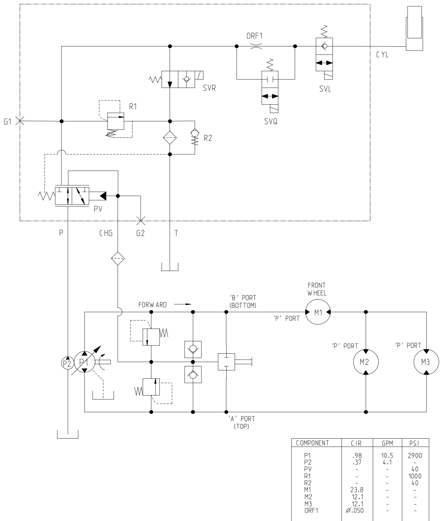
Schema idraulico (Rev. A)
