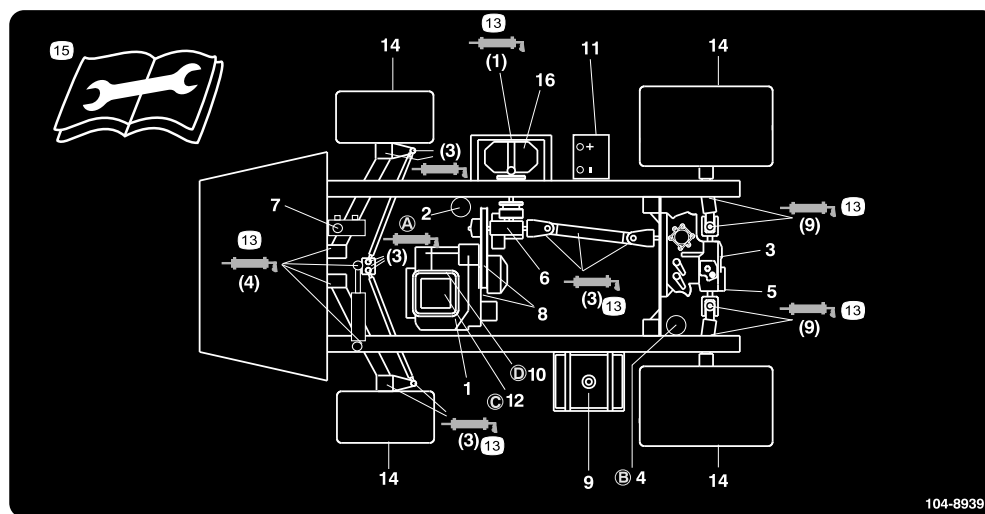
Bild 33 Wartungsstellen
