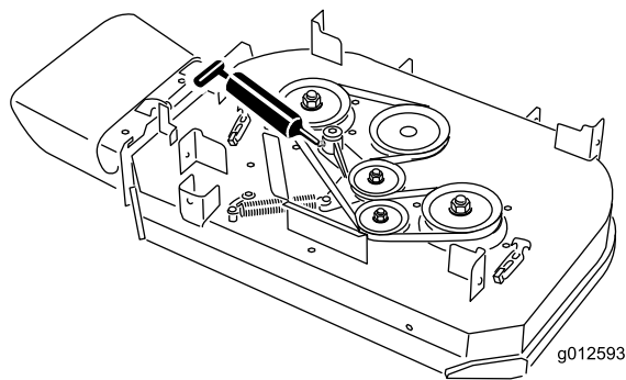
Figura 36 Plataforma de corte de 36 pulgadas (91 cm)
