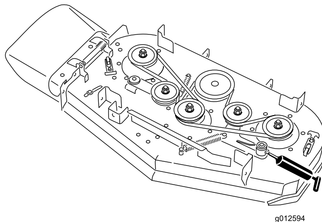
Figura 37 Plataforma de corte de 40 pulgadas (102 cm)
